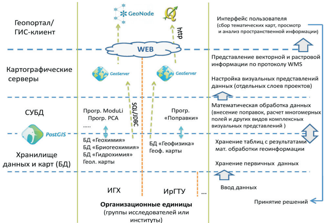
Рис. 4. Архитектура распределенной инфраструктуры пространственных данных для обеспечения геолого-геофизических исследований
