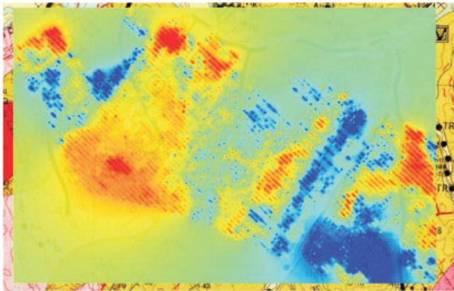
Рис. 2. Пространственное представление робастного главного компонента № 1 на территории Апрельковской РМС
