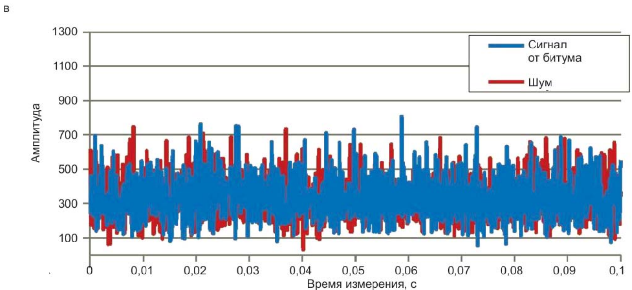
Рис. 8. Пирограммы битумов и образцов пород базеновской (а) и тутлеймской (б) свит (Пальяновская площадь): а – по данным В. Н. Меленевского, ИНГГ СО РАН; в – релаксационные кривые ЯМР сигнала от образца битума, представленного на предыдущем снимке, и шума (по [4])
